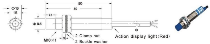
Chart 38 LJ10A3-2-□
