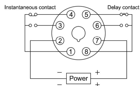
DH48S-2ZH
