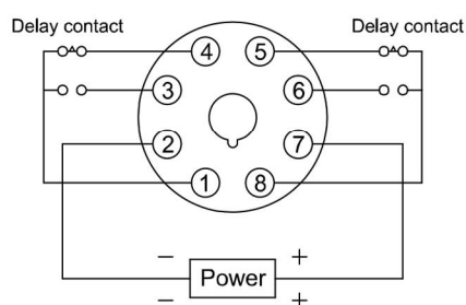
DH48S-S-2Z, DH48S-2Z
