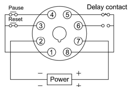
DH48S-S, DH48S-1Z
